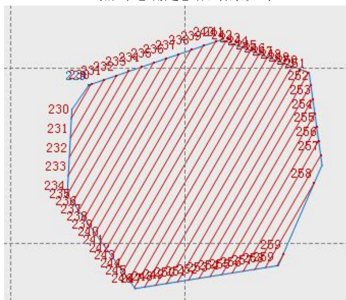
图 5-12 区域布线效果
