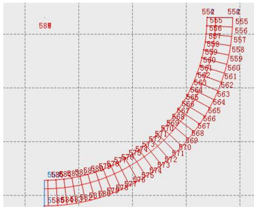
图 5-18 扇形布线效果
