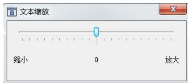
图 7-8 文本缩放
