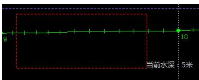
图 9-5 删除水深点
