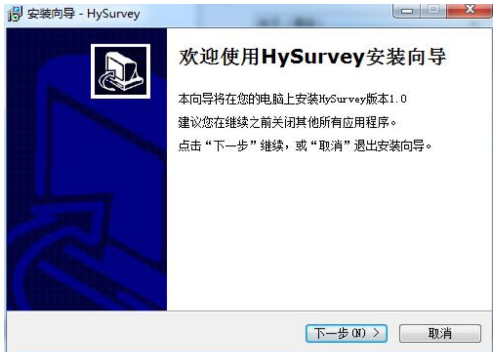
图 1-2 安装向导
