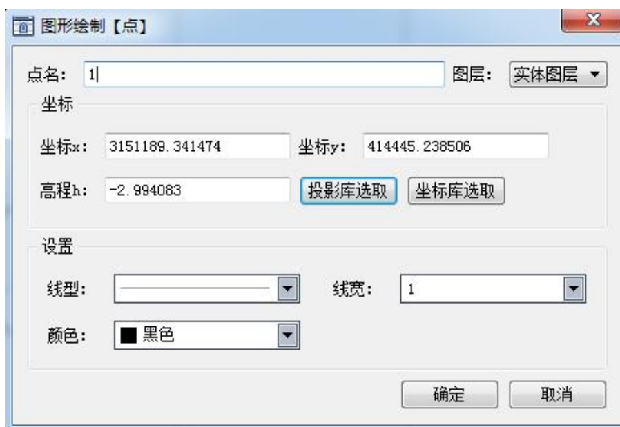
图 5-1 点的绘制
