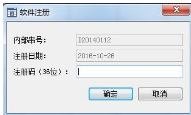
图 10-2 软件注册
