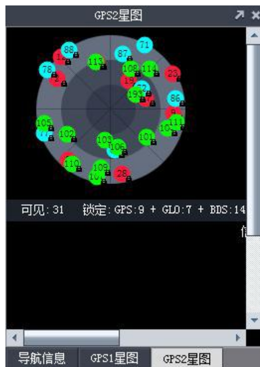
图 11-2 GPS2 星图
