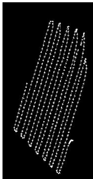
图 9-17 轨迹导出
