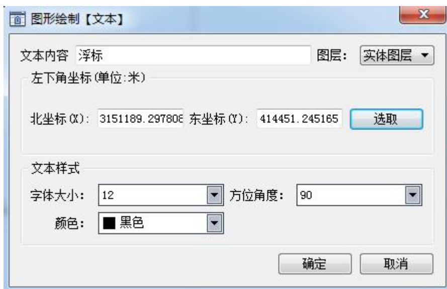
图 5-6 文字注释
