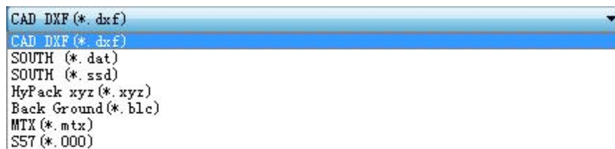
图 3-15 导入图形
