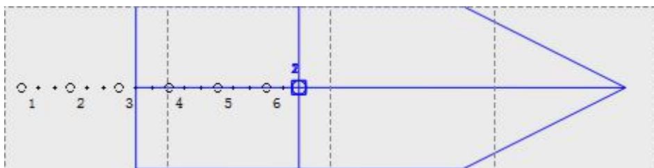
图 7-3 显示测量点
