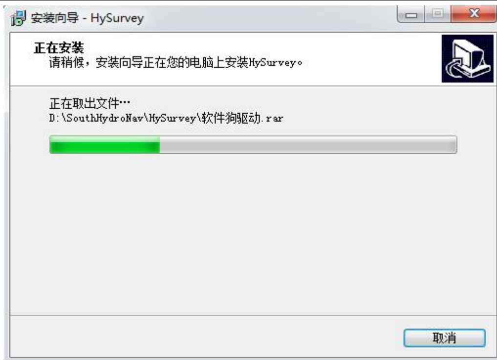
图 1-7 安装界面
