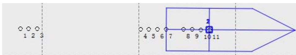
图 4-8 续原来点名
