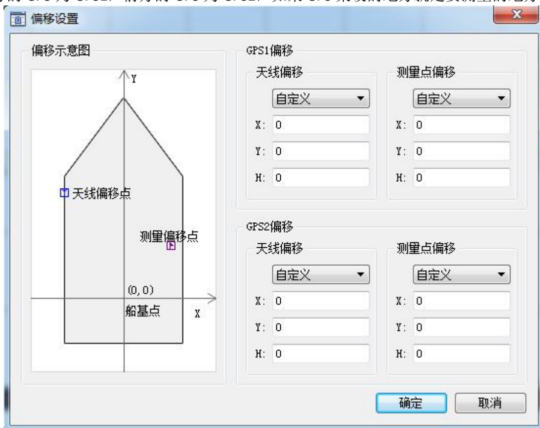
图 4-20 偏移设置
