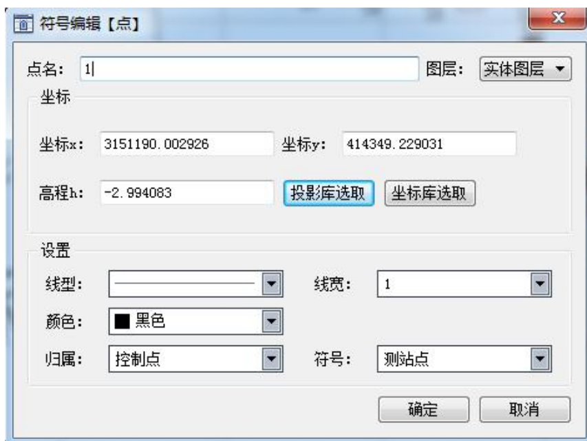
图 5-7 绘制点符号
