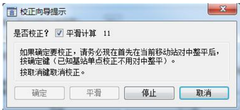
图 4-18 平滑校正
