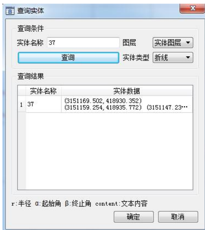
图 4-29 查询实体
