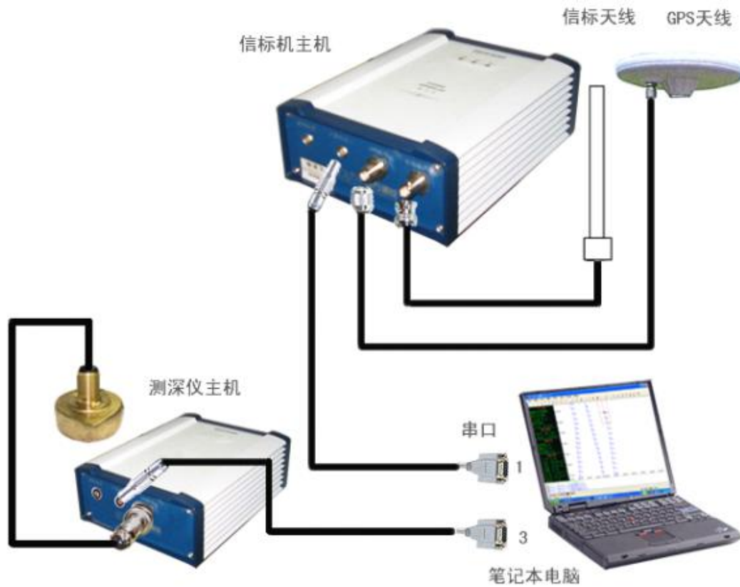
图 2-1 分离式 GPS 连接图
