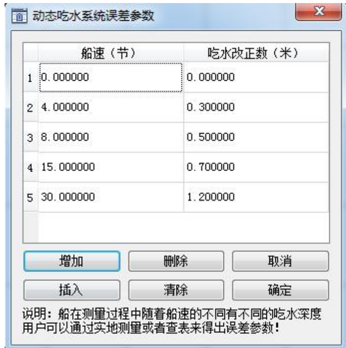
图 9-11 动态吃水改正
