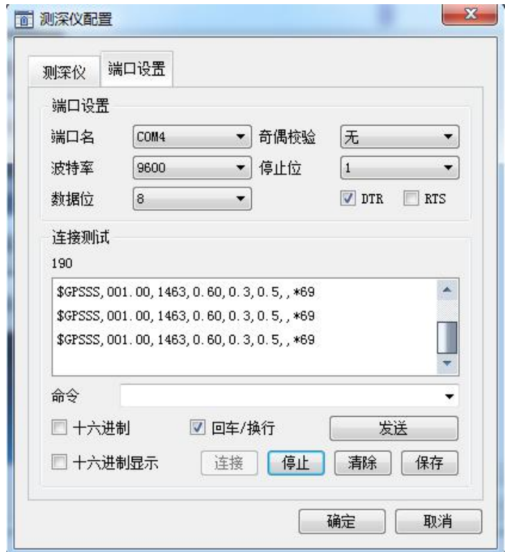
图 3-10 测深仪连接测试
