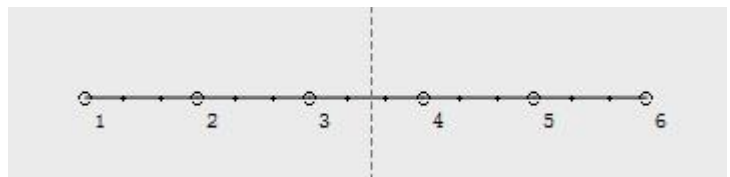
图 7-6 轨迹连线
