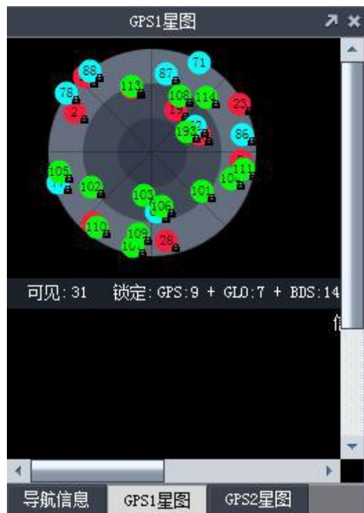
图 11-2 GPS1 星图
