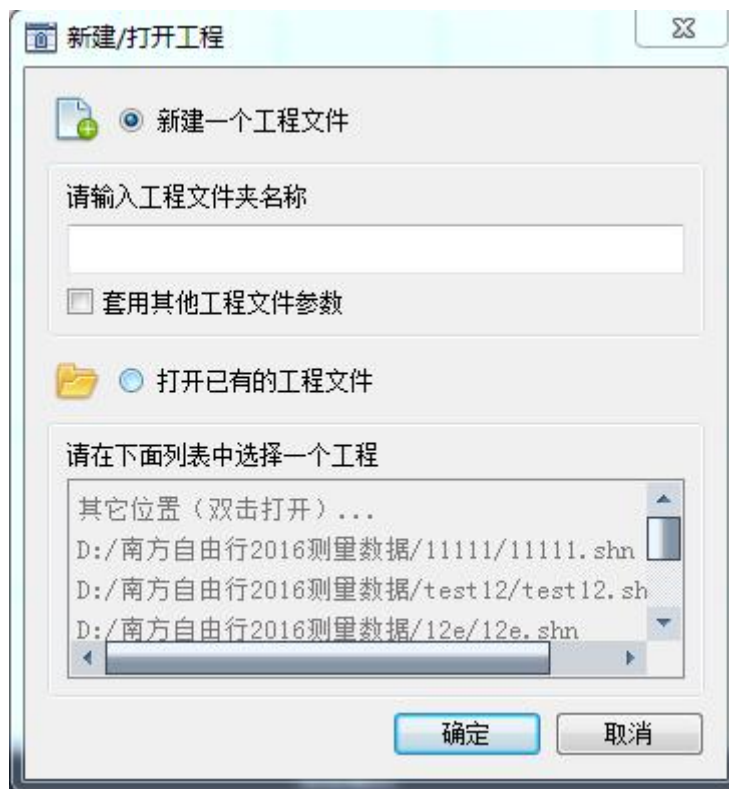
图 3-1 新建工程
