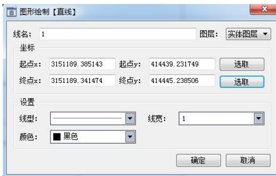
图 5-2 直线的绘制
