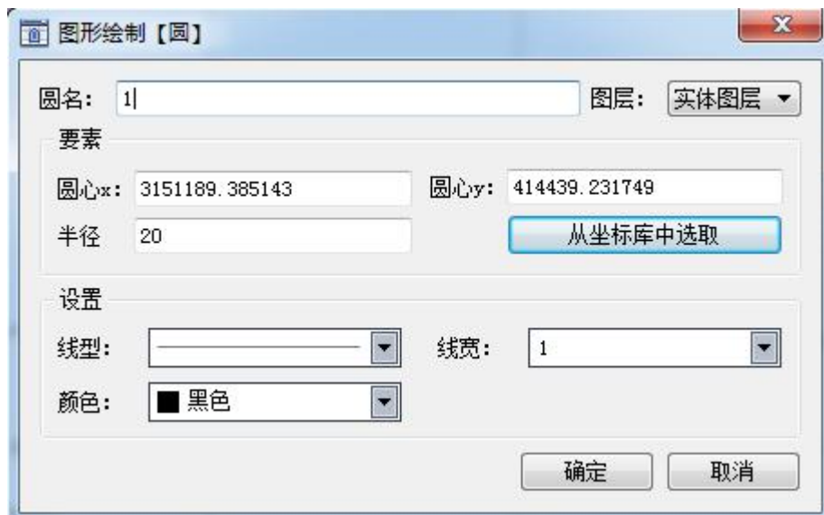
图 5-3 圆的绘制
