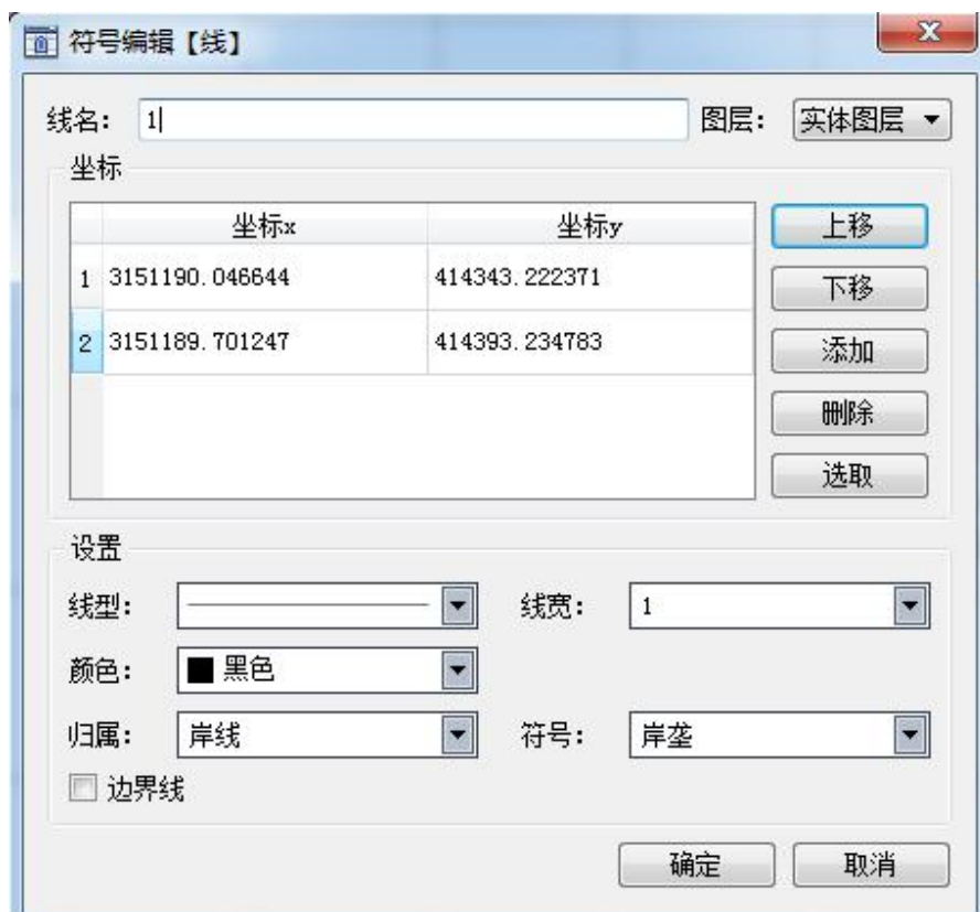
图 5-8 绘制线符号
