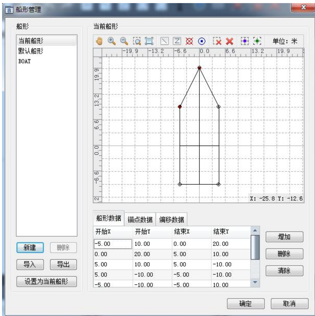
图 5-19 船形设计
