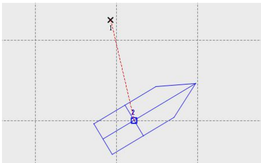
6-2 点放样界面
