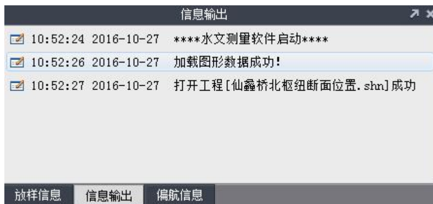
图 11-3 信息输出
