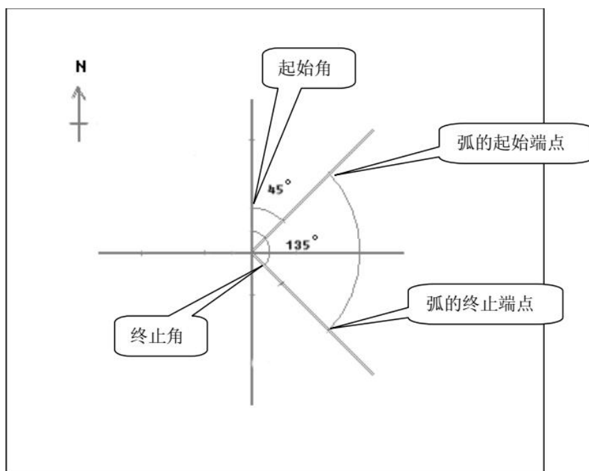
图 5-5 圆弧的定义
