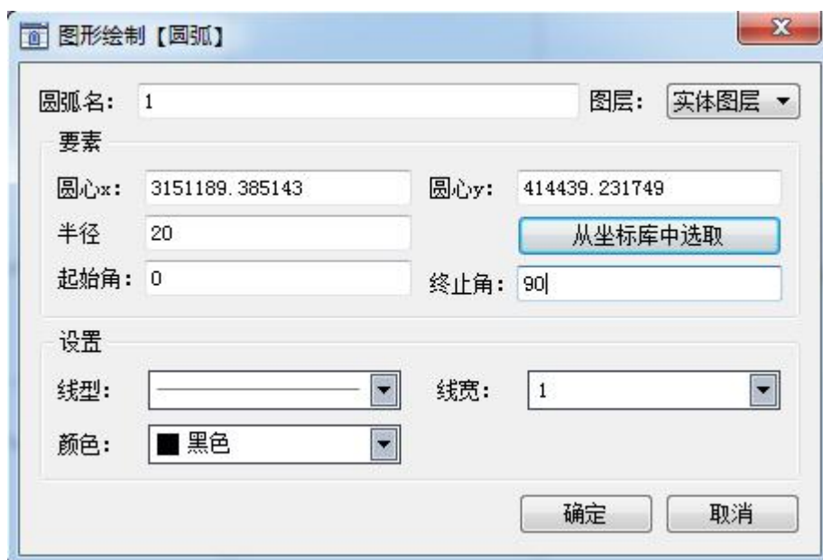
图 5-4 圆弧的绘制
