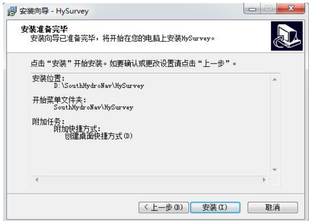
图 1-6 安装
