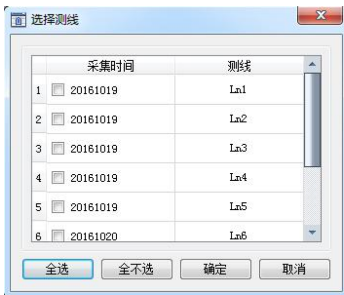
图 8-12 导入测量点
