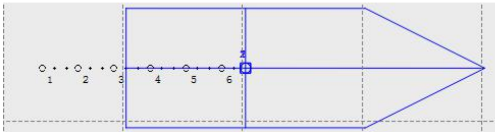
图 7-2 显示轨迹点
