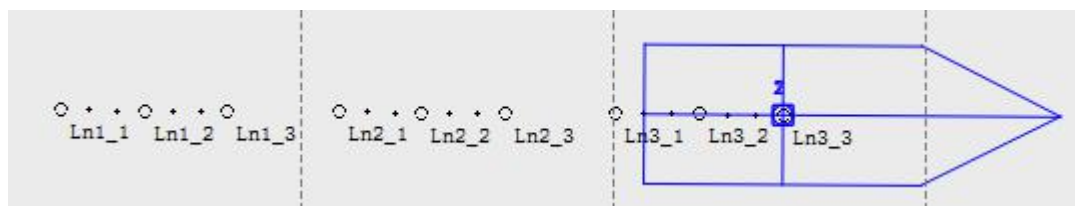
图 4-9 测线+点名
