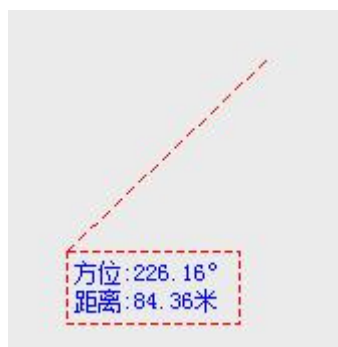
图 8-3 方位角距离
