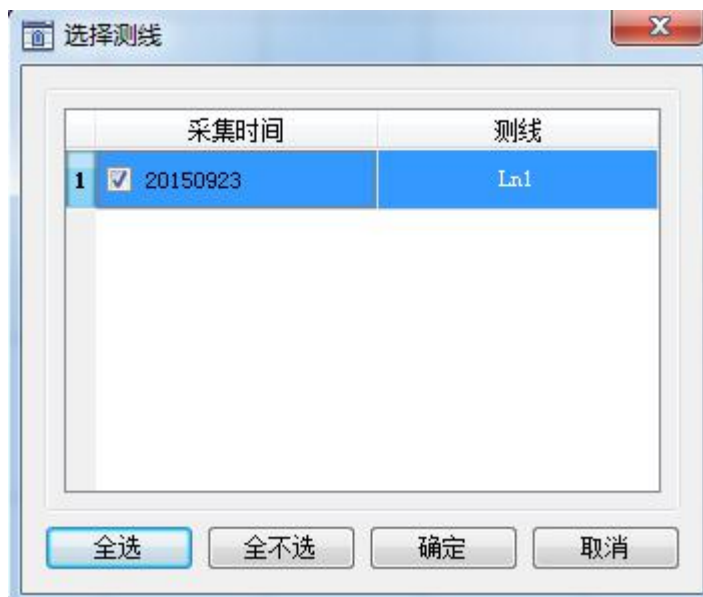
图 9-16 测线选择
