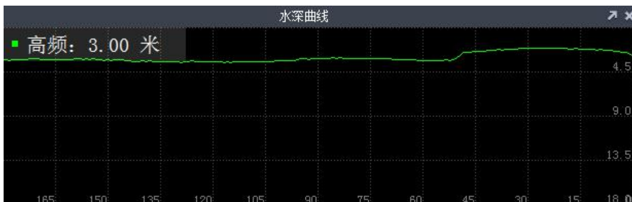
图 11-6 水深曲线
